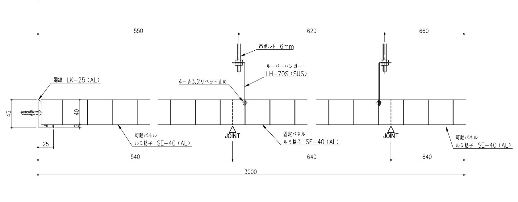
(A) 断面詳細図
