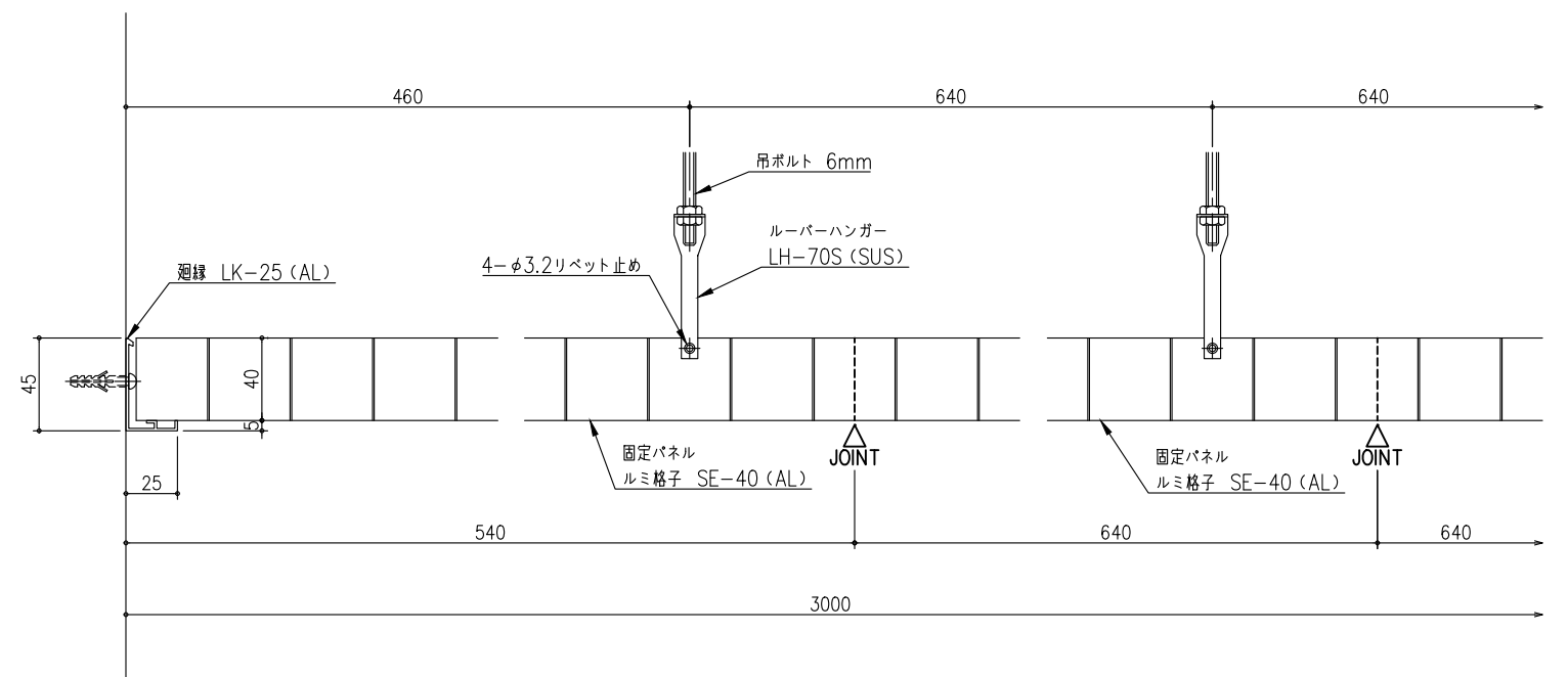
(B) 断面詳細図
