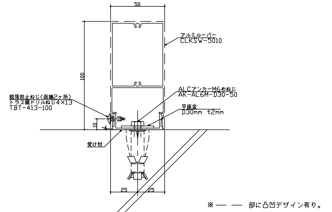
ALC納まり図
