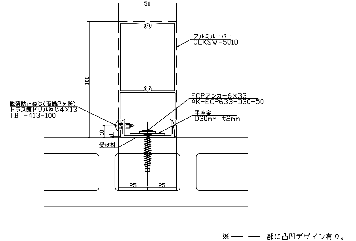
ECP納まり図
