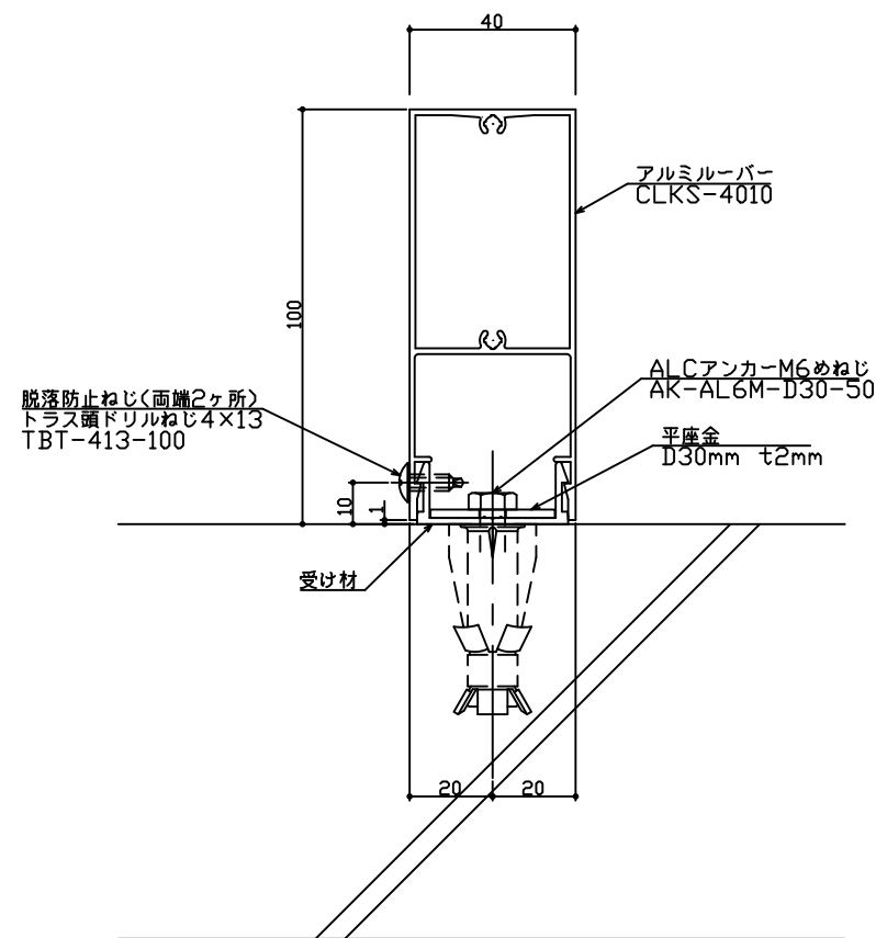
ALC納まり図
