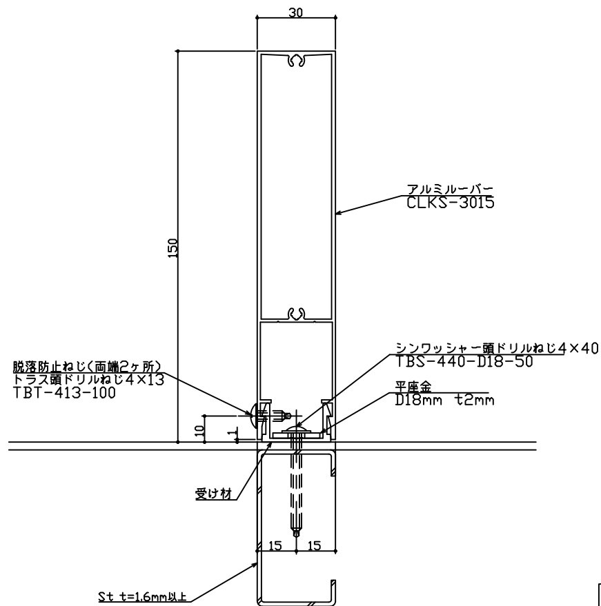
鉄骨納まり図
