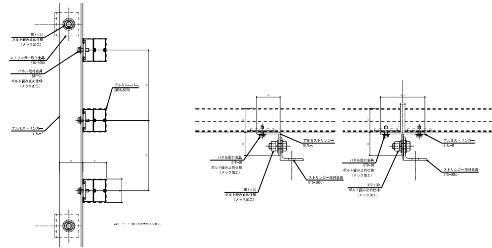
アルミルーバー SHSM-5050 アルミストリンガー STAL-7 STAL-8
