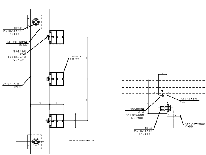
アルミルーバー SHSM-5050 アルミストリンガー STAL-13
