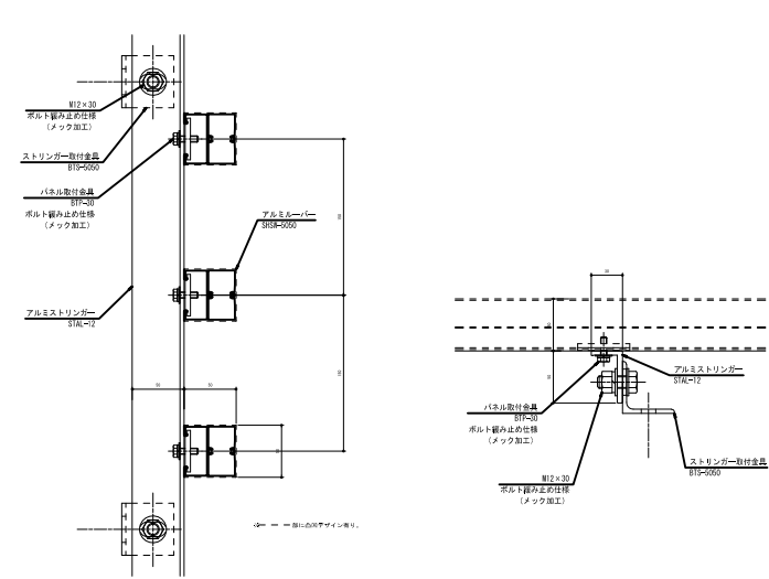
アルミルーバー SHSM-5050 アルミストリンガー STAL-12
