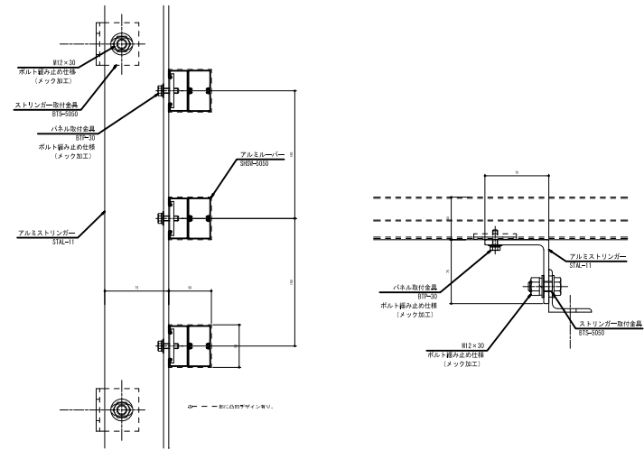
アルミルーバー SHSM-5050 アルミストリンガー STAL-11
