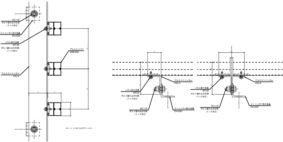
アルミルーバー SHSM-5050 アルミストリンガー STAL-5 STAL-6
