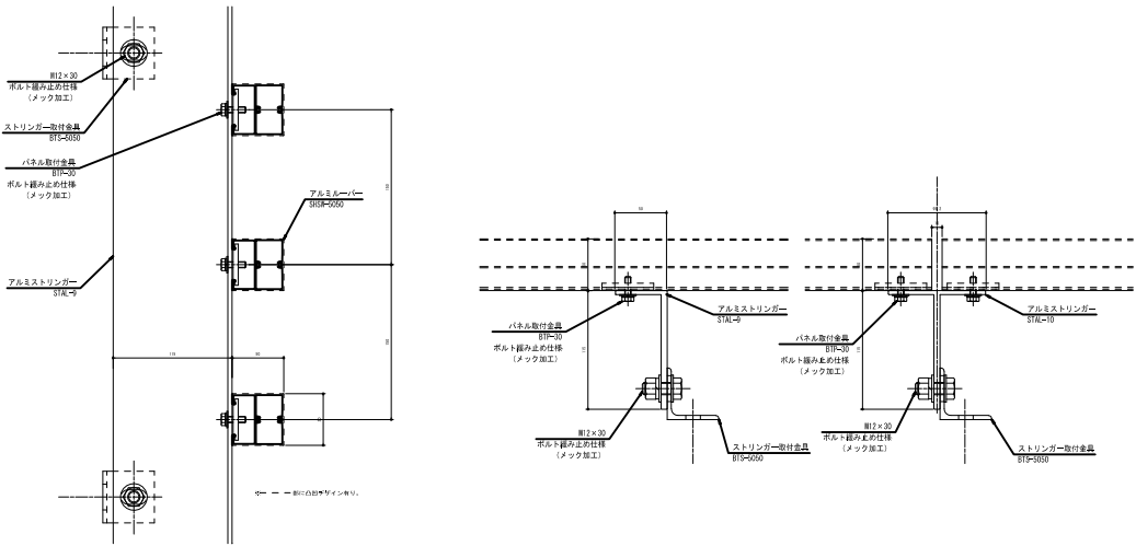
アルミルーバー SHSM-5050 アルミストリンガー STAL-9 STAL-10
